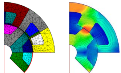
有限要素法による静磁場解析
